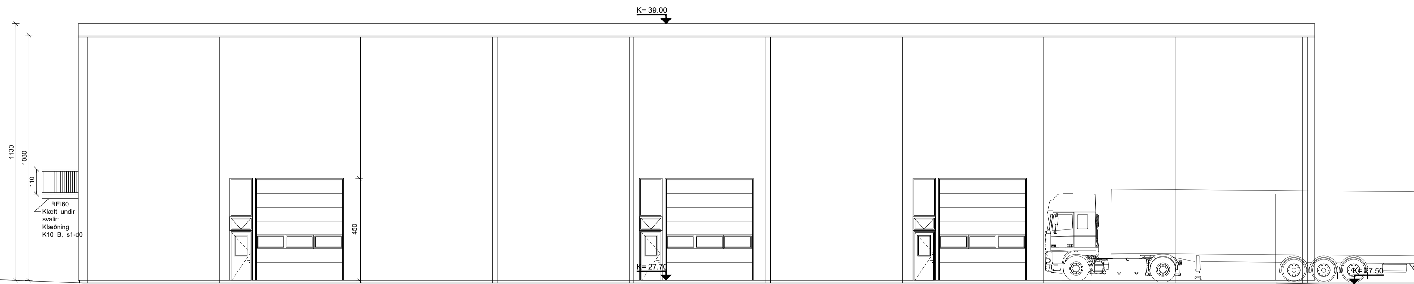
Útlit Norður Mkv: 1:100
