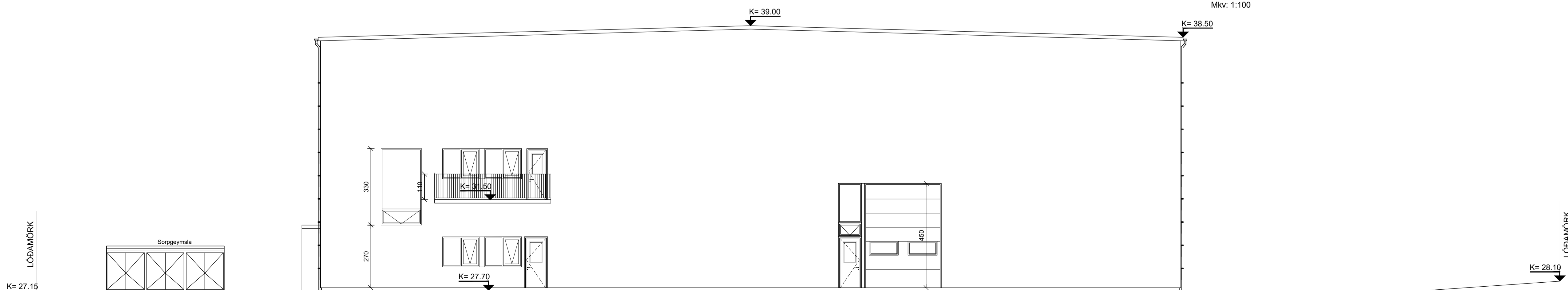
Útlit Austur Mkv: 1:100
